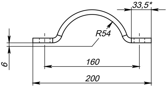
Поз.4 (Полухомут)
