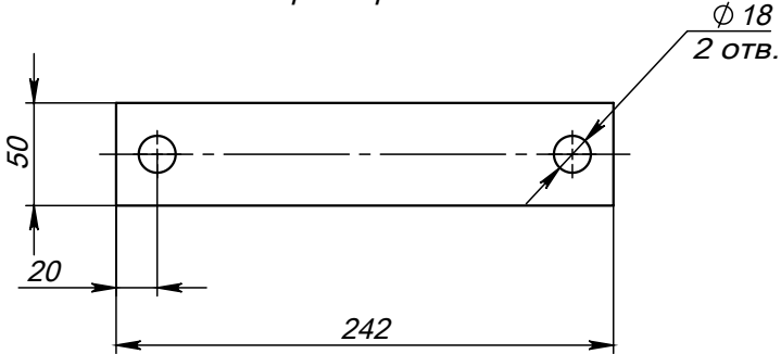
Поз.4 (Полухомут) развертка
