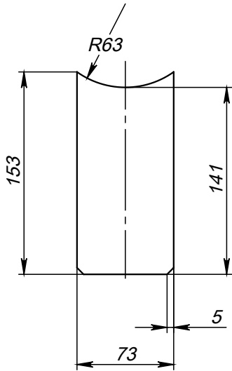
Поз.3 (Ребро)
